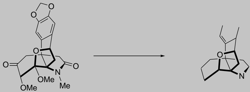
(+)-periglaucine C ( 3 )
